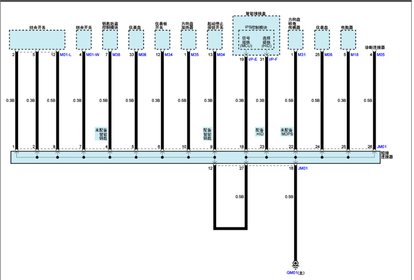
搭铁分布(1)
